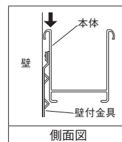
側面図
